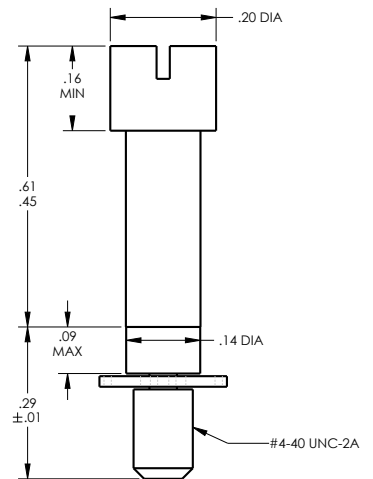
#4/40 DCJS100S
