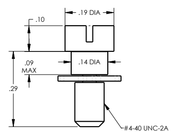
#4/40 DCJS100SLP
