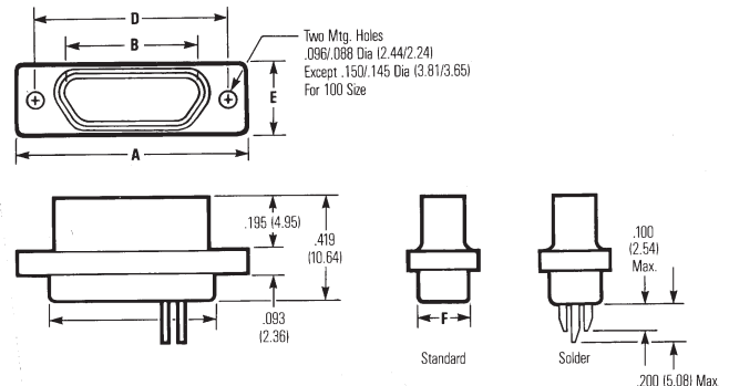
Socket
