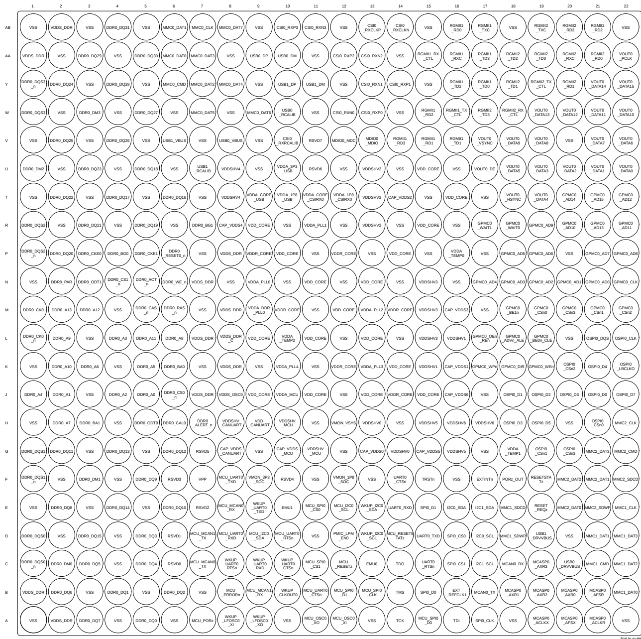
Figure 6-1. AMB FCBGA-N484 Pin Diagram (Bottom View)
