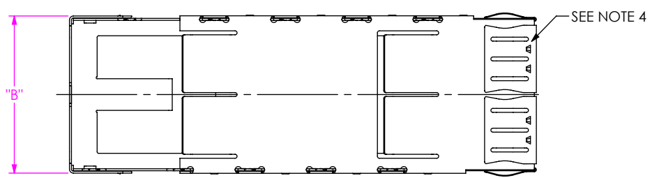
FIG 1 QSFP-C-1-1-S-F SHOWN
