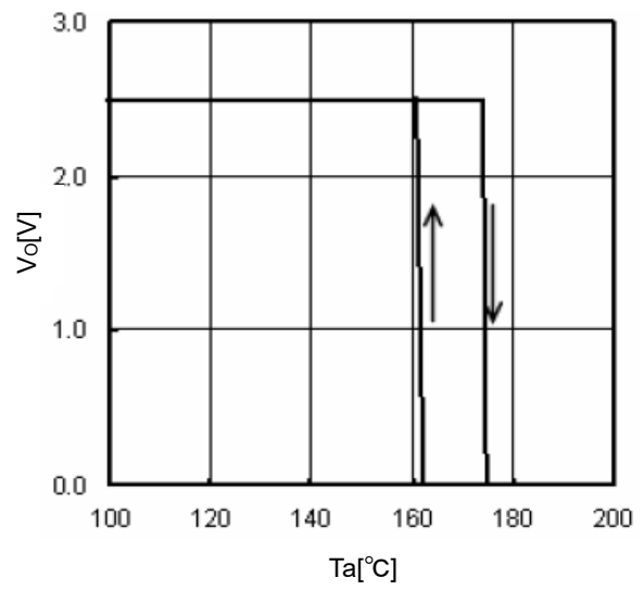
Fig.28 TSD
