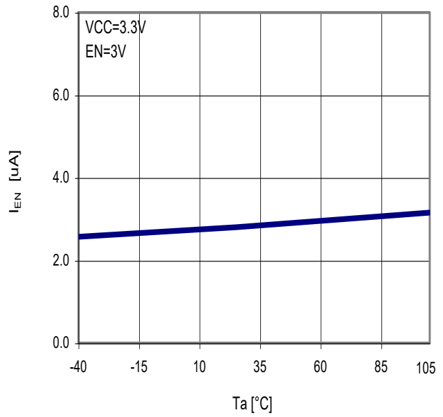
Fig.24 T_a - I_{EN}
