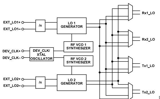
Figure 362. RF LO
