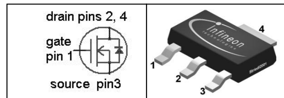
PG-SOT223
