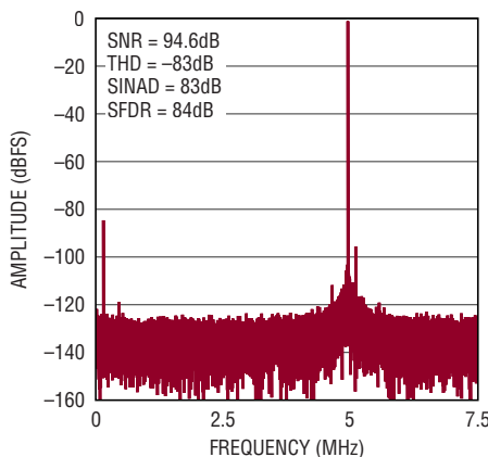
32k Point FFT f_{SAMPL} = 15\text{Mpsps} , f_{IN} = 5\text{MHz}
