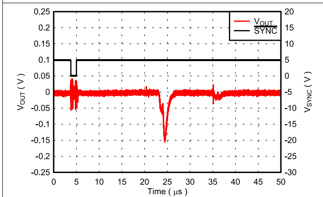
DAC range: \pm 20\text{ V}
