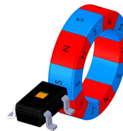
Figure 8-8. ZX Outer Edge 2
