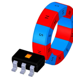
Figure 8-10. ZY Outer Edge 1
