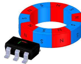
Figure 8-6. XY Outer Edge 2
