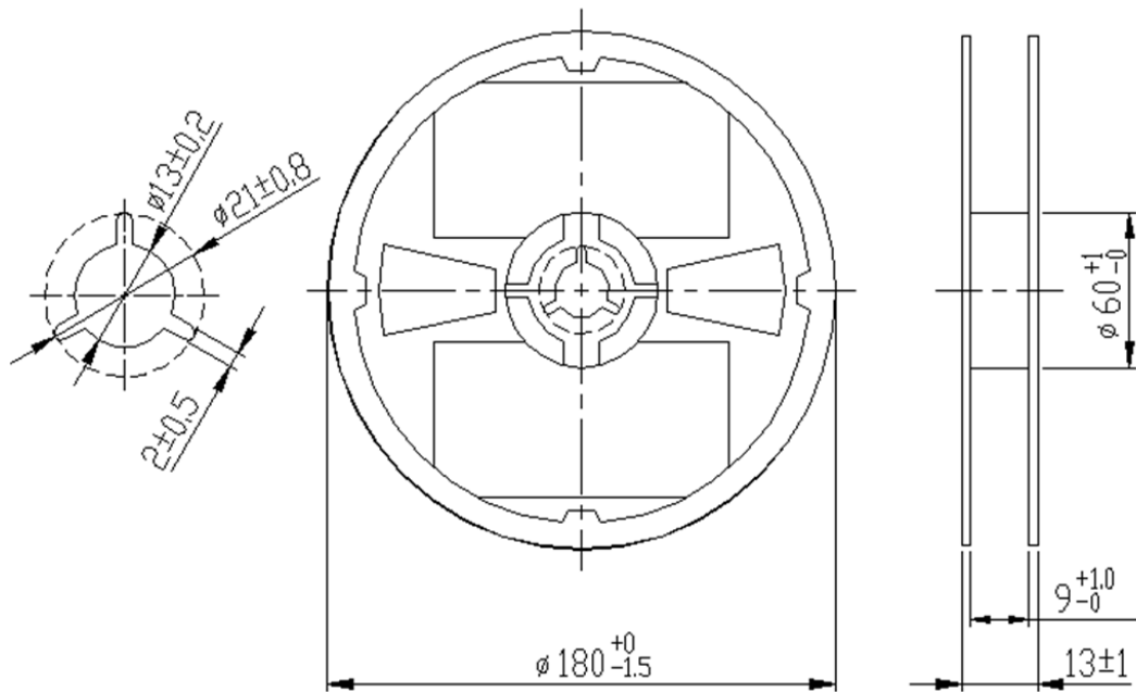
Reel Dimensions
