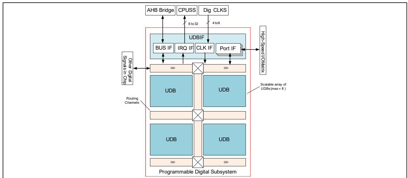
Figure 6 UDB Array
