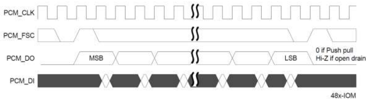
Figure 66: IOM Format
