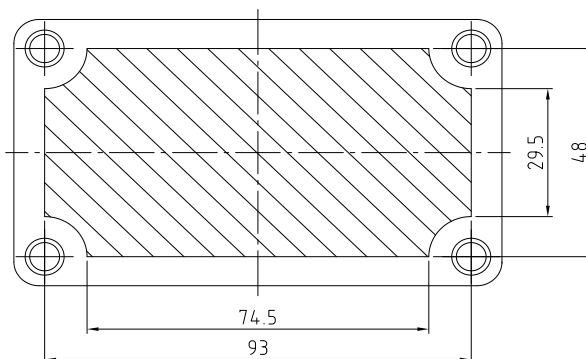
Sperrfläche für Thermisches Interface Material restricted area for Thermal Interface Material
