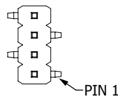
SMT, Pin 1 Right (D) Only Even Positions
