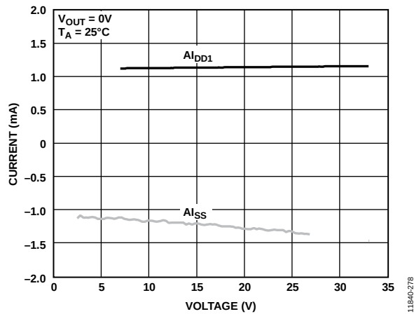
Figure 70. I DD1 /I SS Current vs. AV DD1 /|AV SS | Supply
