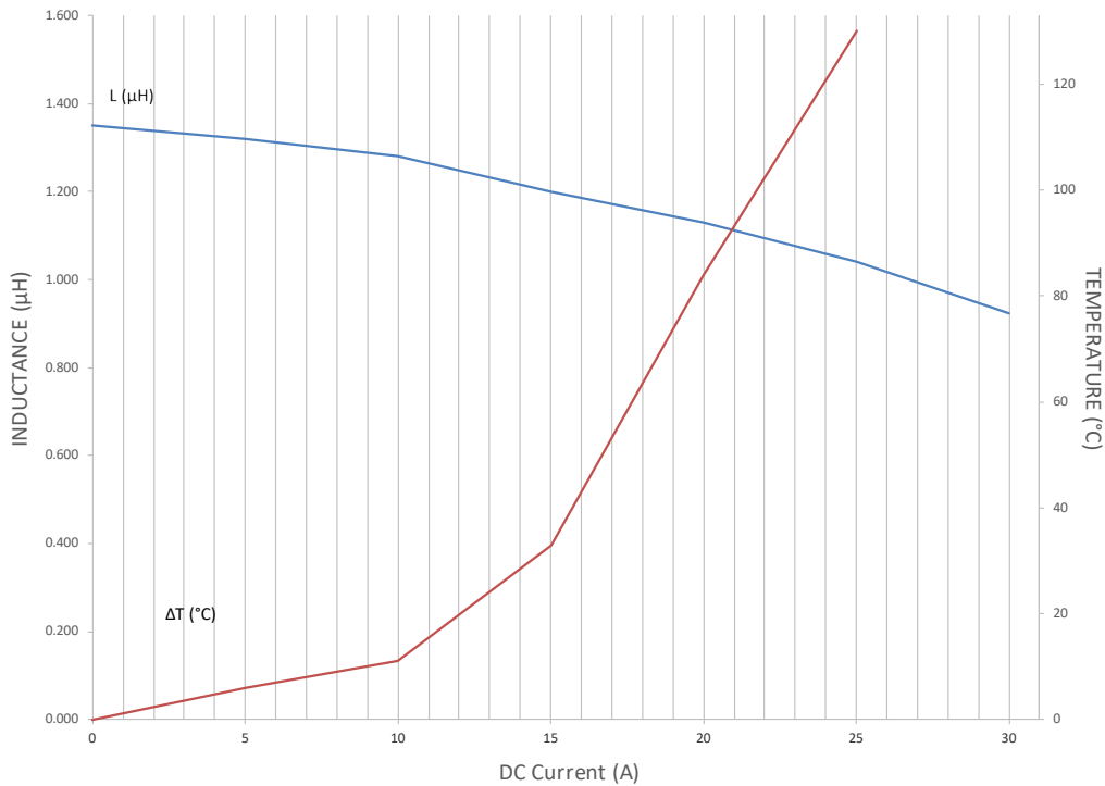
I&T Curve
