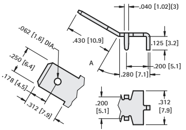
.250 (6.4) TAB
