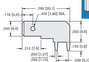
.250 (6.4) TAB
