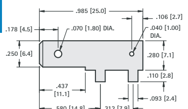
.250 (6.4) TAB
