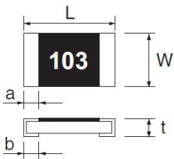
■MCR004/006/01/03
