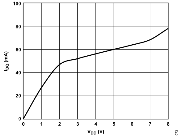
Figure 72. I DQ vs. V DD , R BIAS = 1.43 kΩ
