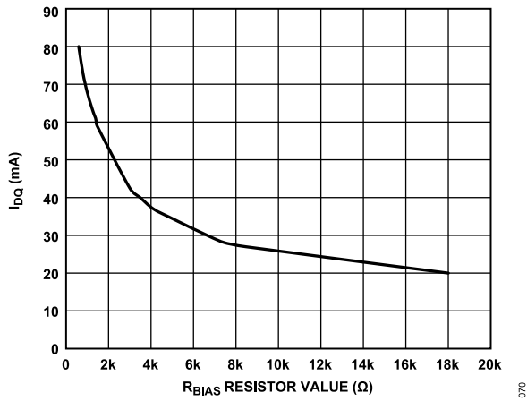
Figure 70. I DQ vs. R BIAS Resistor Value, V DD = 5 V
