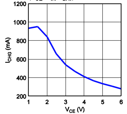
Thermal Protection ( V_{CE}=V_{IN}-V_{BAT} )
