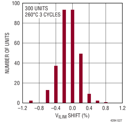
V_{ILIM} Shift Due to IR Reflow
