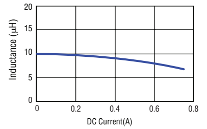
SRN2010TA-100M
