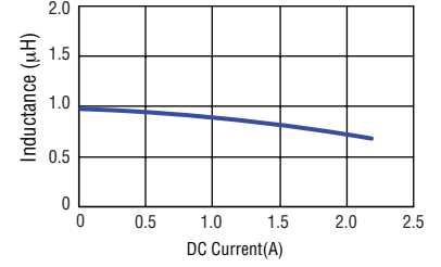
SRN2010TA-1R0Y
