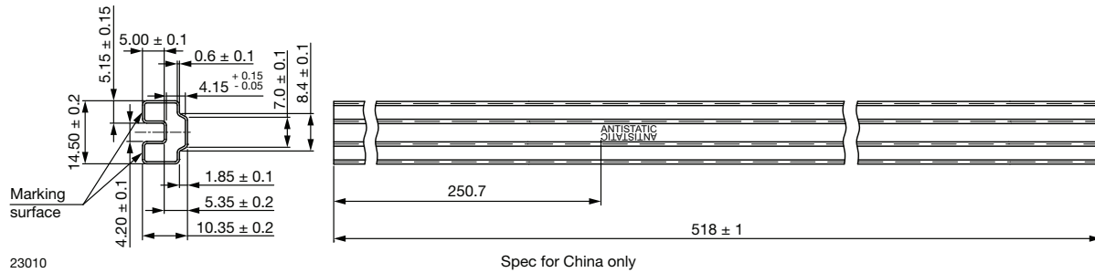
Fig. 16 - DIP-6
