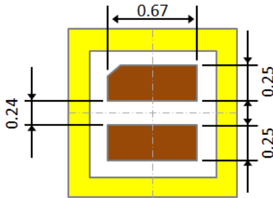
<Chip Pad>
