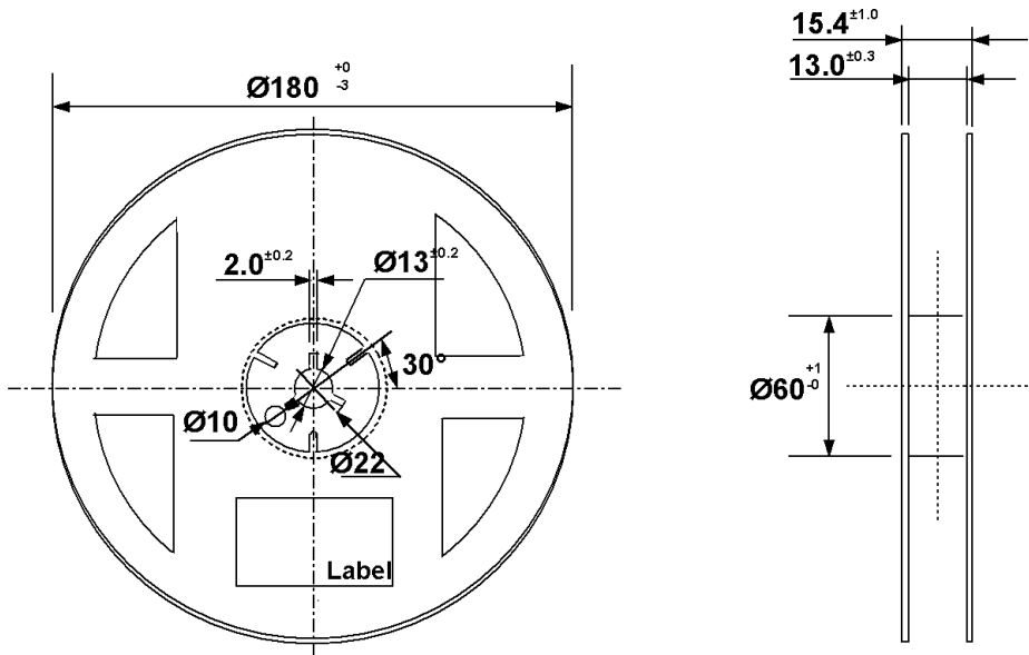
Tolerance ±0.2 , Unit:mm
