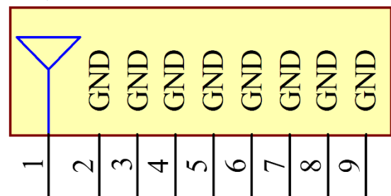
TAOGLAS_SGGP.18.4.A.08 ANT1
