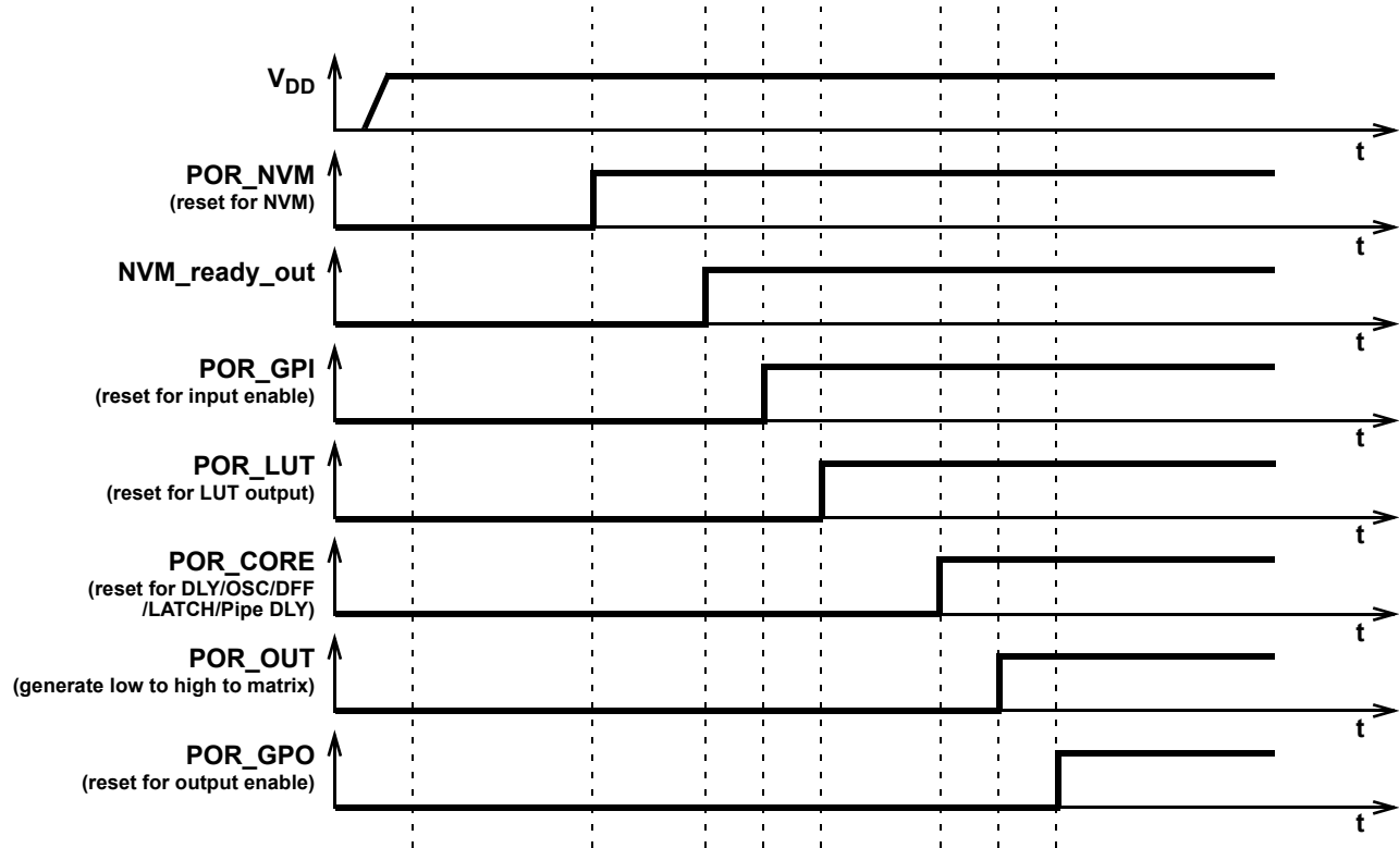
Figure 87: POR Sequence
