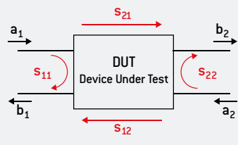
Figure 2: S parameters
