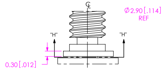
DETAIL 'G' SCALE 8 : 1
