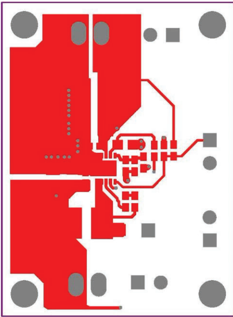
Fig. 23 - Top Layer
