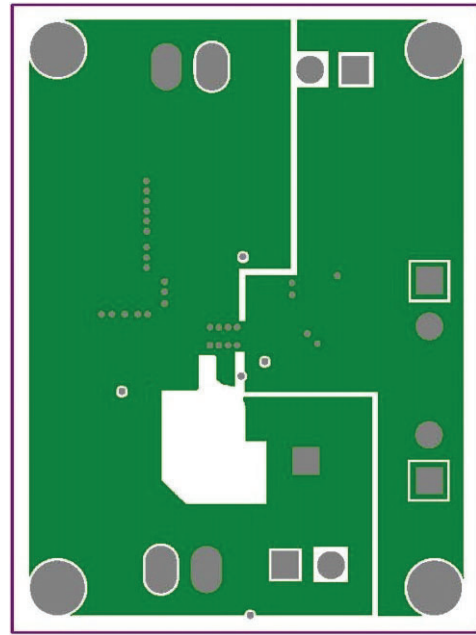
Fig. 25 - Inner Layer 1
