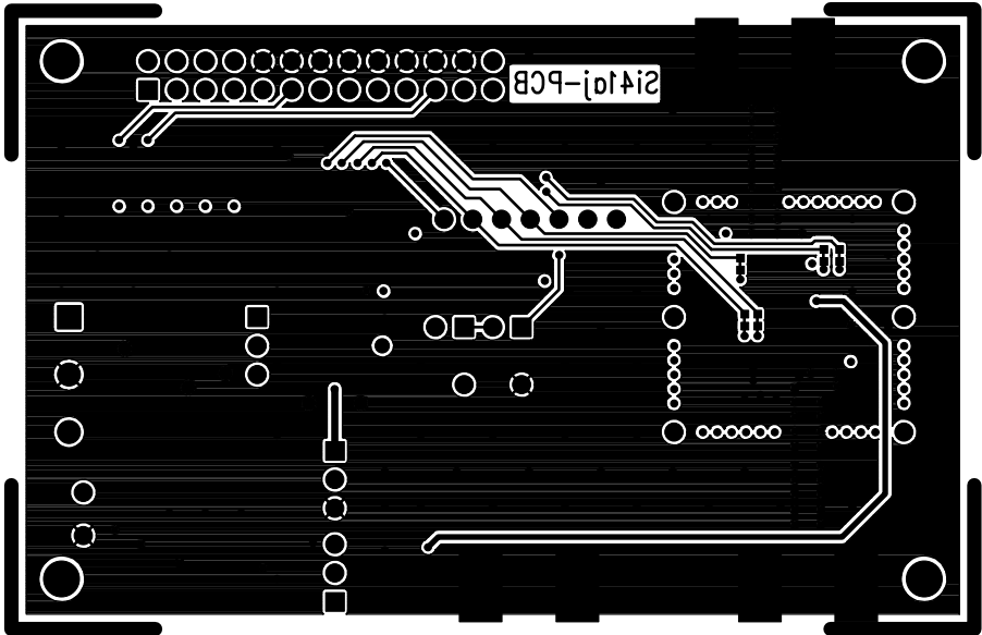
Figure 27. Si4133BT Solder
