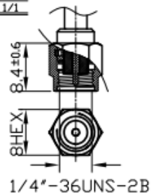
SMA(M) ST DETAIL : 'B' SCALE: 1/1
