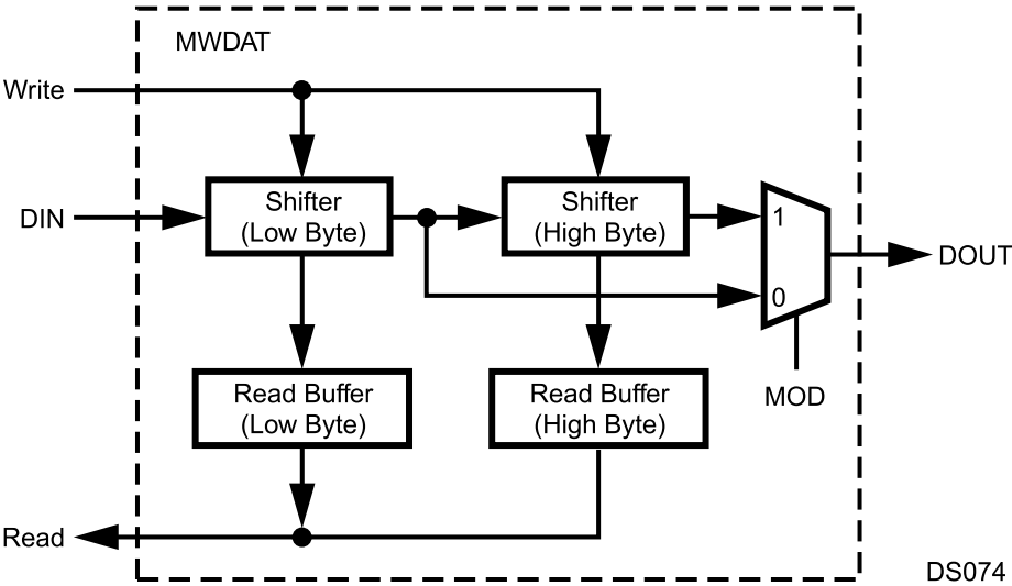
Figure 23-8. MWDAT Register
