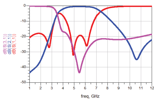
RFDIP2012050LQT
