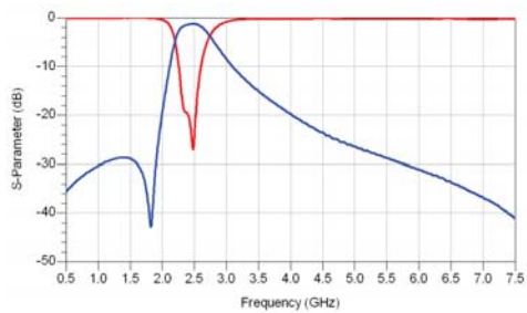
RFBPF2012080AC2T00
