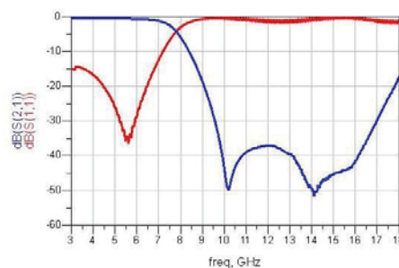
RFLPF1608060Y08Q1C
