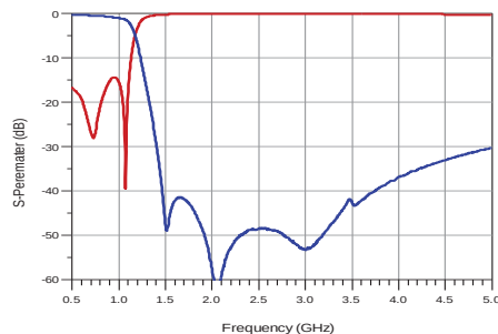
RFLPF1608060Y18Q1C
