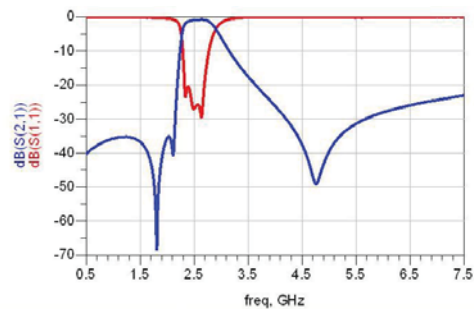
RFBPF2012080AGT
