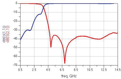
RFLPF2012100F18Q1C
