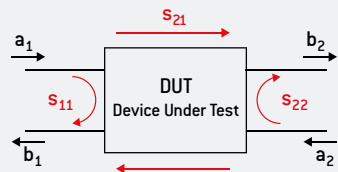
Figure 2: S parameters
