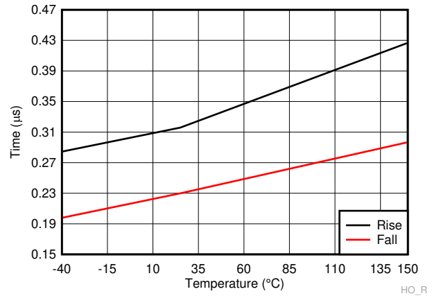
A. C_L=100nF
