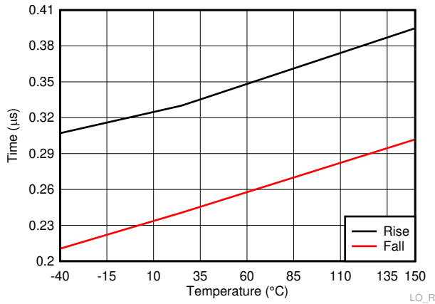
A. C_L=100nF
