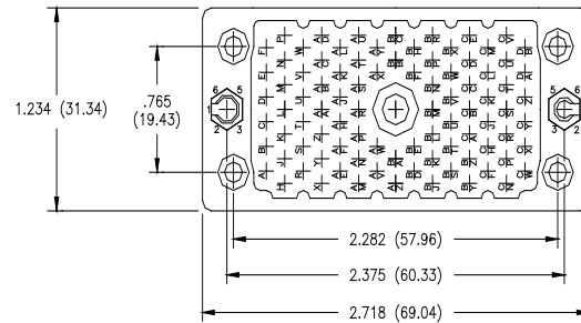
120 PIN RECEPTACLE
