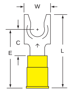
SS-33-14-NB 1/4 12-10
