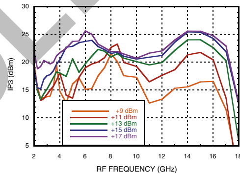
Input IP3 vs. LO Power, IF = 1500 MHz
