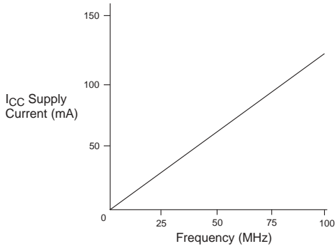
EPF10K10A
